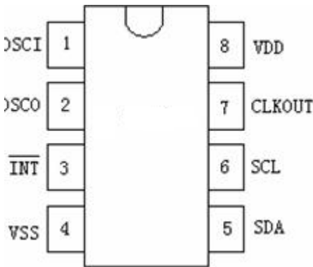
图 3. 引脚图
