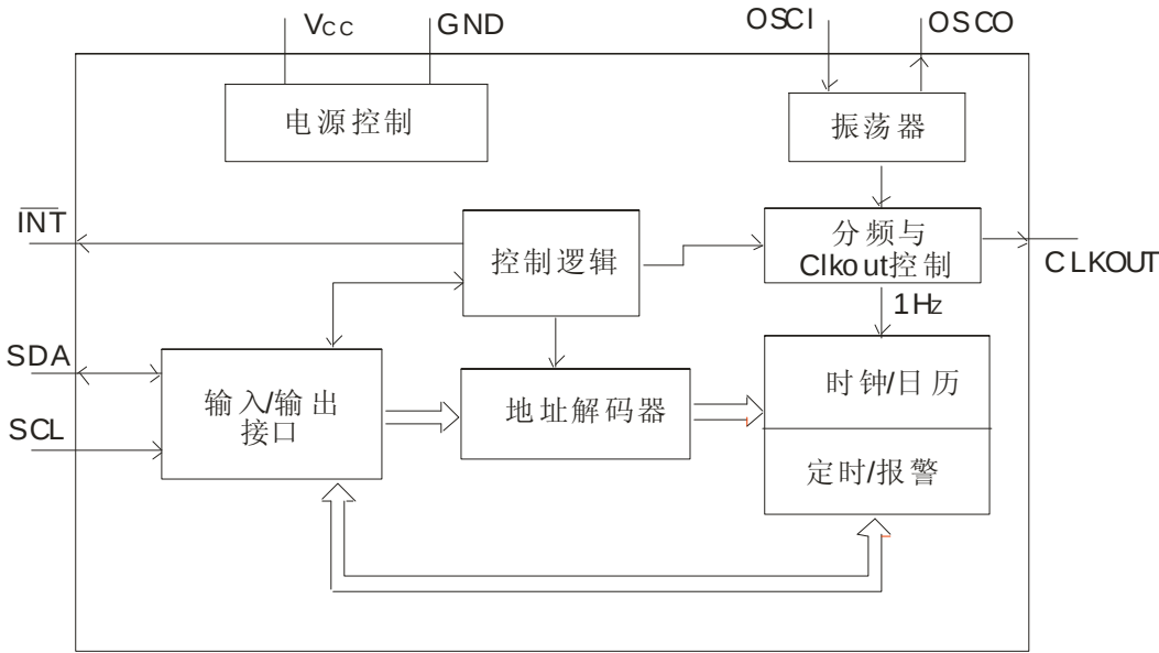
图 2. 方框图
