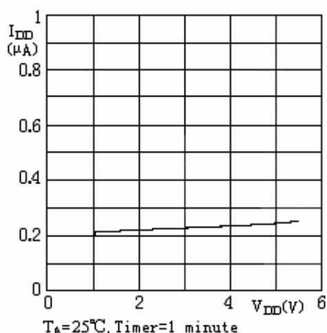
CLKOUT禁止时, I_{DD} 与 V_{DD} 的关系图-
